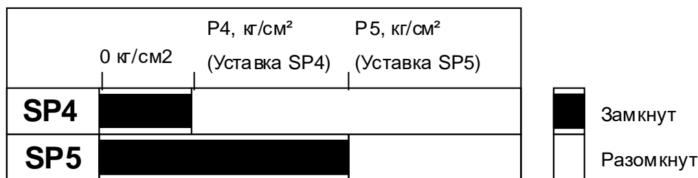
Рисунок 8.2 – диаграмма состояния контактов датчиков.
