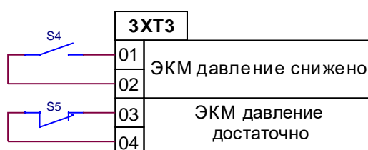
Рисунок 8.1 – схема подключения датчиков НП.
